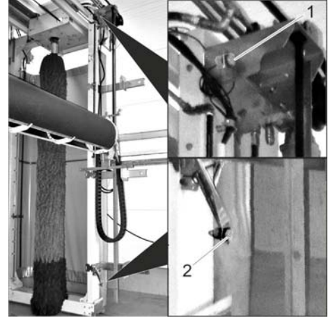
صورة 7 1. المفتاح الحدي لكمرة سقف الضغط العالي بأعلى (HdO) 2. المفتاح الحدي لكمرة سقف الضغط العالي بأسفل (HdU)
