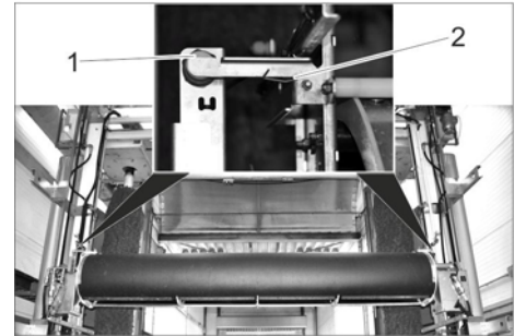
صورة 8 1. المفتاح الحدي لمفتاح أمان كمرة سقف الضغط العالي 2. نابض
